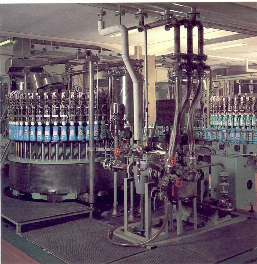
柔軟仕上剤ハミグの自動充填ライン
