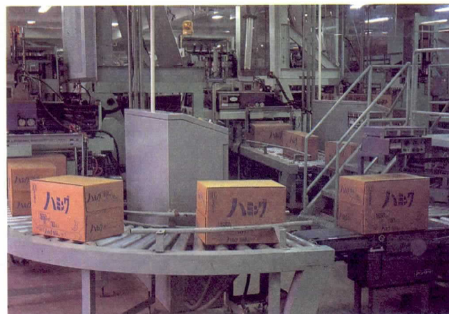
自動倉庫へのコンベアライン
