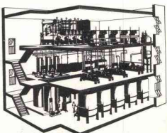
完成したシャープレス高速度自動練石鹼製造装置
