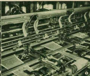
編立工場のフルファッション機の細部。24台のうち12台が最新式の米国産。その精密さで15D、20Dの細い糸1本のまま靴下が編まれる。1足分4000米。
