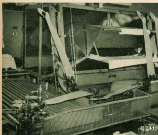
乾燥機。プロクター式とボイラー式があるが出来上った製品は型にはめて乾燥機に入れられ乾燥の後最終検査、マーク押し、取合せ、包装で市場におくられる。
