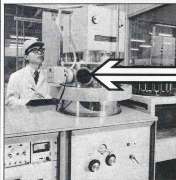
▲電子コーティング(プラズマ)を施すスパッタリング装置
